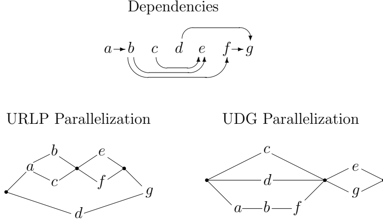
Fig. 10. Example parallelizations using URLP and UDG.
